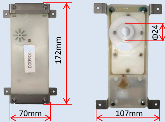
①スマートセンサ取付治具セット品（標準5台/セット）
